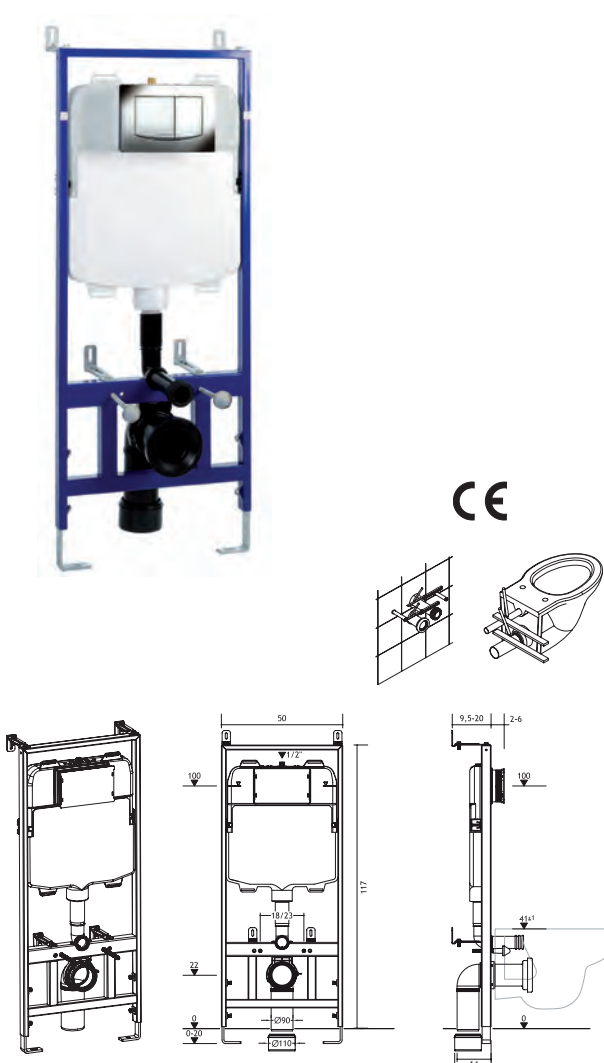
Cisterna empotrada con bastidor para WC suspendido al suelo. Placa doble pulsador incluida Concealed cistern with frame for floor-standing WC. Dual push plate included. Réservoir encastré avec bâti pour wc au sol. Plaque double poussoir.
