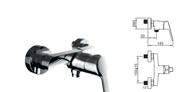
Mezclador para ducha. Shower mixer. Mitigeur douche
