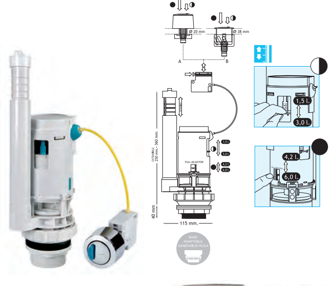
Descarga eco-control con cable. Water saver cable flushing valve. Décharge éco-contrôle à câble.
