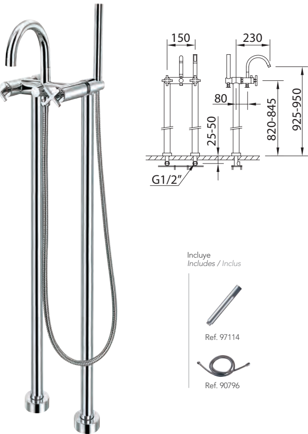
Baño ducha fijación suelo, aireador, inversor. Floor standing bath-shower mixer, aerator, diverter. Mélangeur bain-douche sur colonne avec prise d'eau au sol, aérateur, inverseur automatique
