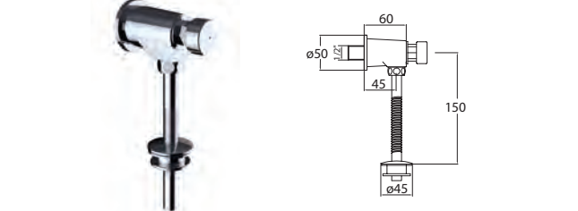
Grifo mural de 1/2" para urinario, 7 segundos, cartucho M28. Urinal 1/2", 7 seconds, cartridge M28. Robinet temporsié urinoir 1/2", 7 secondes, cartouche M28.
