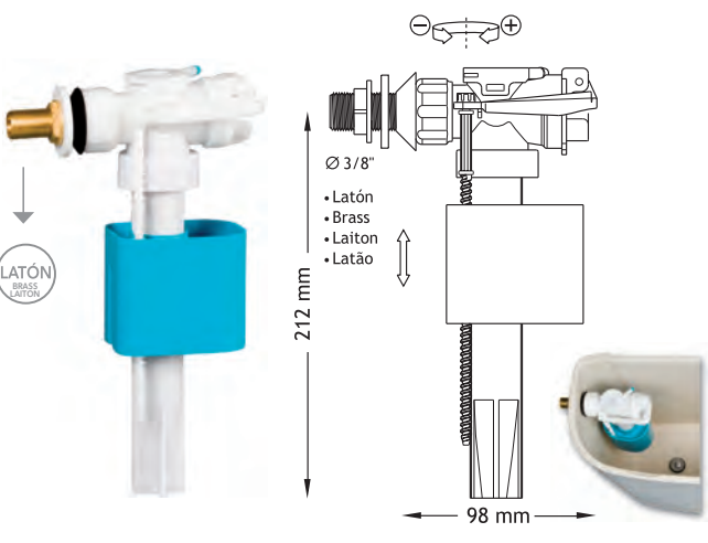
Válvula alimentación lateral. Silencioso, rápido y compacto. Side fill valve. Silent, quick and compact. Arrivée d'eau latérale. Silencieux, rapide et compact.
