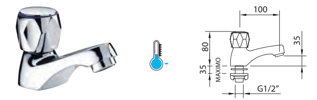
Grifo de repisa, con aireador, índice de agua fría. Deck mounted single basin faucet, with aerator, cold water indice. Robinet lavabo, aérateur.
