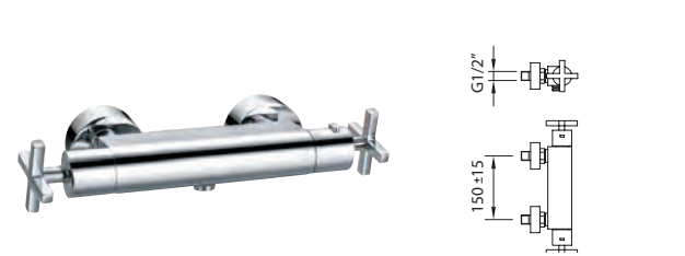
Mezclador para ducha. Shower mixer. Mélangeur douche thermostatique, aérateur, inverseur
