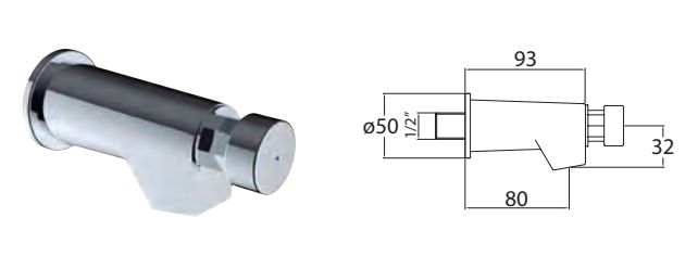
Grifo mural para lavabo, con aireador, <14 segundos, cartucho M28 Wall mounted basin tap, with aerator, <14 seconds, cartridge M28 Robinet simple, avec aérateur, <14 secondes cartouche M28
