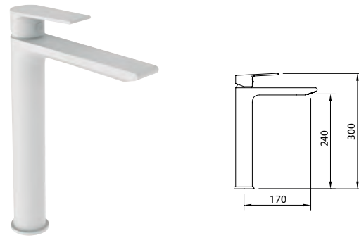
LAVABO 240 BLANCO MATE Matte white tall basin mixer 240 / Mitigeur lavabo blanc mat 240
