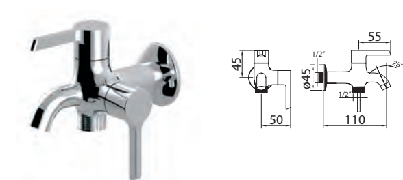
Grifo de pared salida fregadero / lavadero / lavadora. Wall mounted single tap. Robinet, aérateur
