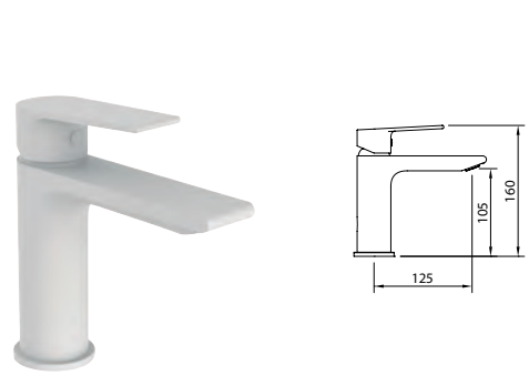
LAVABO 105 BLANCO MATE Matte white tall basin mixer 105 / Mitigeur lavabo blanc mat 105
