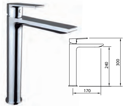
LAVABO 240 / Basin mixer 240 / Mitigeur lavabo 240
