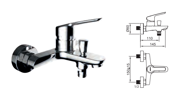
Mezclador con aireador baño-ducha, inversor automático. Bath-shower mixer with aerator, automatic diverter. Mitigeur bain-douche, aérateur, inverseur automatique
