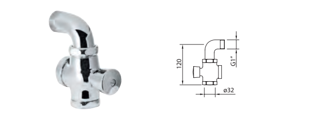
Fluxor exterior para urinario. Urinal external fluxor. Robinet temporsié urinoir mural.
