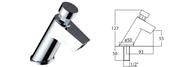
Grifo de repisa para lavabo, con aireador, <14 segundos, cartucho M28 Deck mounted basin tap, with aerator, <14 seconds, cartridge M28 Robinet simple, avec aérateur, <14 secondes cartouche M28
