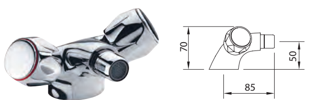
Mezclador con aireador a rótula y flexibles M-10 3/8" x 370 mm. Mixer, swivel aerator, flexible hoses M-10 3/8" x 370 mm. Mélangeur bidet, aérateur rotule, raccords flexibles M-10 3/8" x 370 mm
