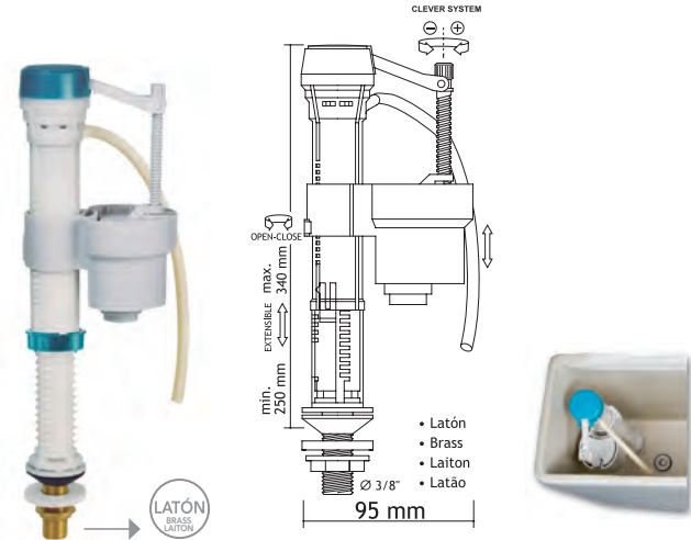
Válvula alimentación inferior. Silencioso, rápido y compacto. Bottom fill valve. Silent, quick and compact. Arrivée d'eau inférieure. Silencieux, rapide et compact.
