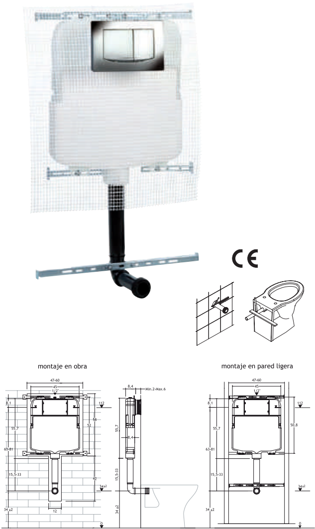
Cisterna empotrada para WC al suelo. Placa doble pulsador incluida Concealed cistern for wall-hung WC installation. Dual push plate included. Réservoir encastré pour wc suspendu ou au sol. Plaque double poussoir.
