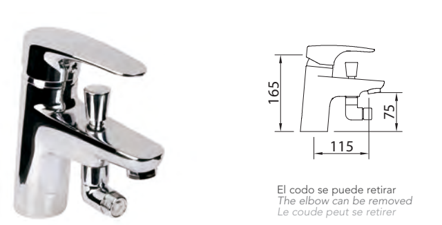
Mezclador baño-ducha, aireador, inversor automático y flexibles M-10 3/8" x 500 mm. Bath-shower mixer, aerator, automatic diverter, flexible hoses M-10 3/8" x 500 mm. Mitigeur bain-douche monotrou, aérateur, inverseur automatique, raccords flexibles M-10 3/8" x 500 mm
