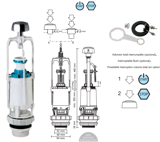
Descarga eco-control interrumpible. Fácil montaje. Volumen total interrumpible (opcional). Water saver press & stop flushing valve. Easy assembly. Interruptable flush (optional). Possibilité d'interruption du vidage du réservoir
