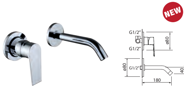
LAVABO EMPOTRADO MURAL Concealed basin mixer / Mitigeur lavabo à encastrer
