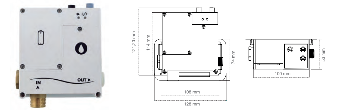
Caja estándar con platina sujeción pared incluida. Para 60739-60740. Standard box with enclosure wall included. For 60739-60740. Boîtier standard avec platine de fixation murale incluse. Pour 60739-60740.
