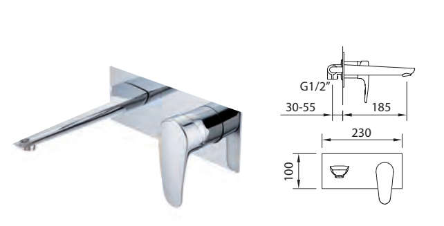
Mezclador empotrable, caño mural con aireador, longitud 185 mm. Concealed basin, aerator, wall mounted spout length 185 mm. Mitigeur lavabo encastré, aérateur, bec 185 mm.
